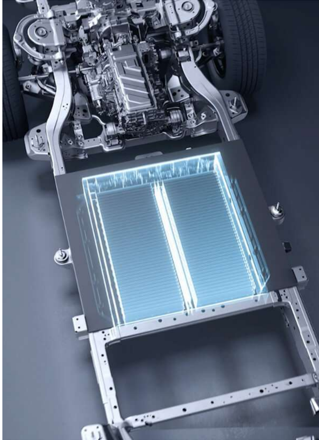
الابتكار تقنية Cell to Chassis تعزز صلابة الهيكل بنسبة ٢٢%.
